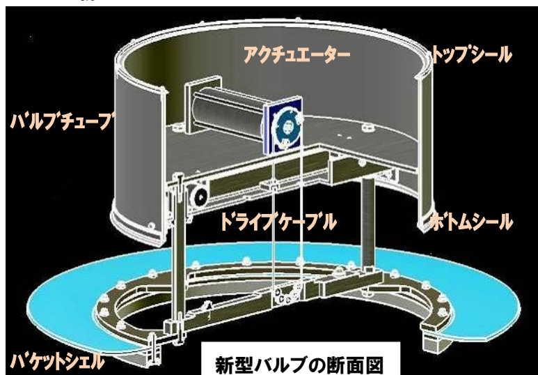
新型バルブ
